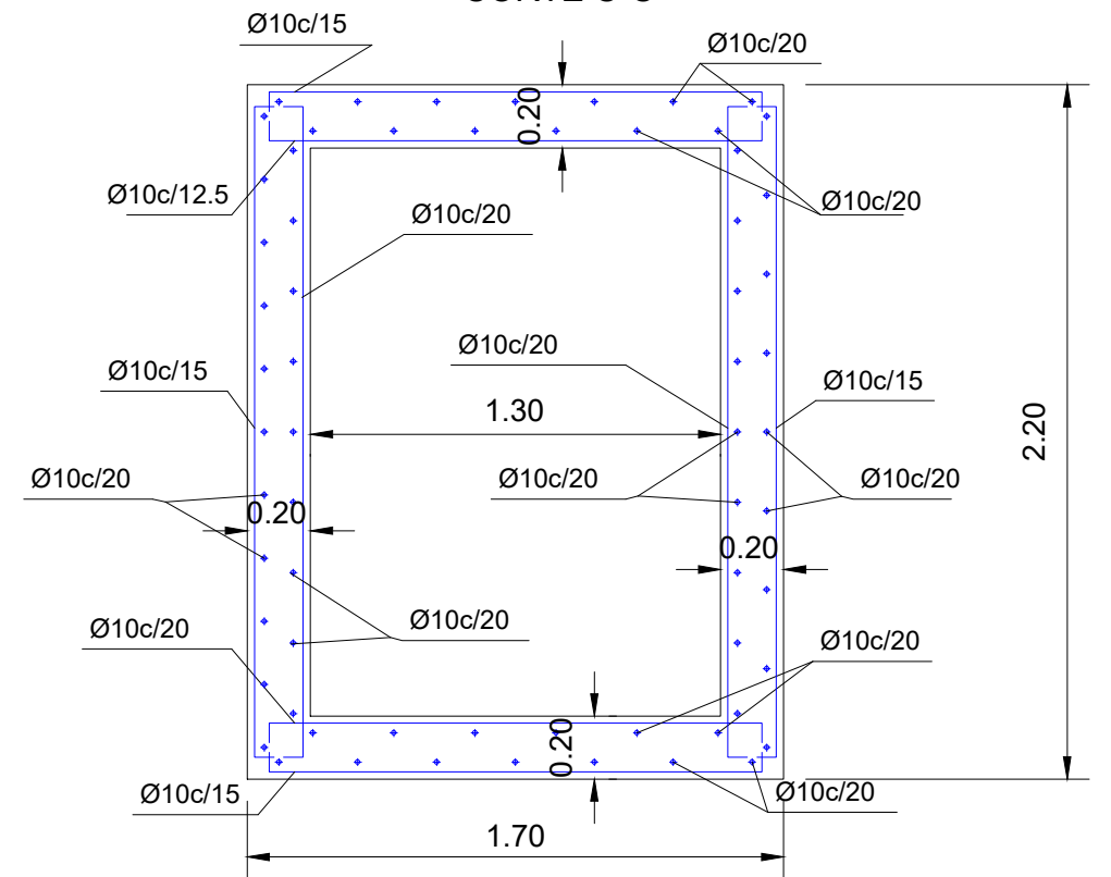
CONDUCTO DE VUELCO CORTE C-C
