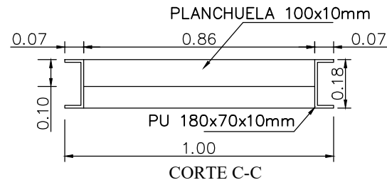
DETALLE MÓDULO DE REJA Esc. 1:20
