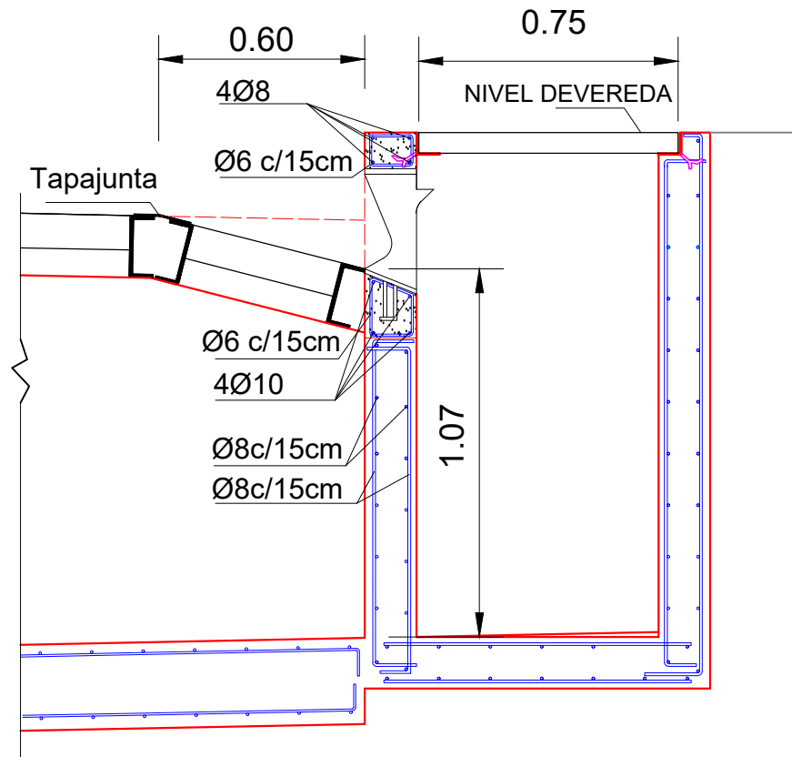
CAPTACIÓN EN ZONA DE REJA Esc. 1:20
