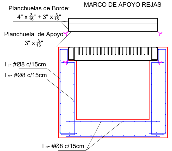
CONDUCTO DE VUELCO CORTE C-C
