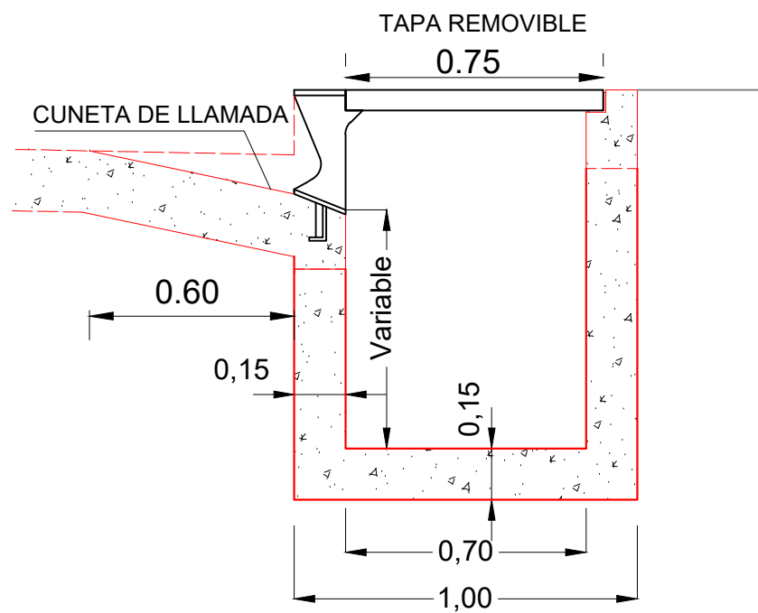
CAPTACIÓN EN ZONA DE IMBORNALES Esc. 1:20
