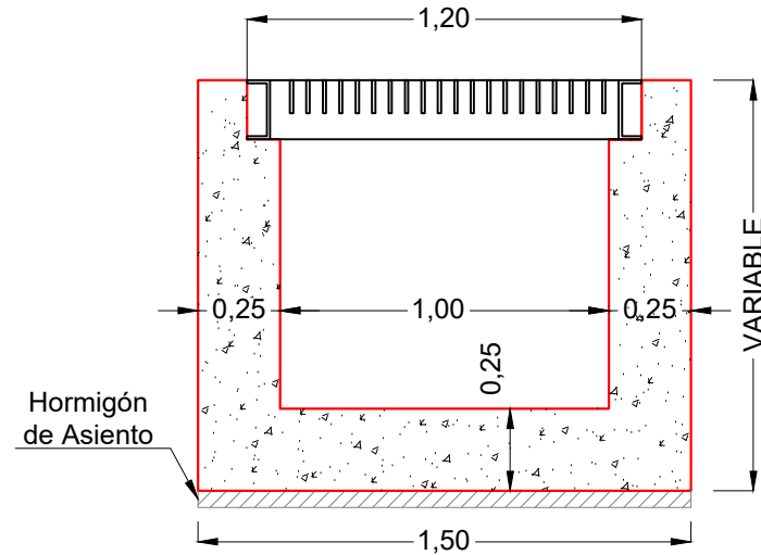
CAPTACIÓN EN ZONA DE REJA Esc. 1:20
